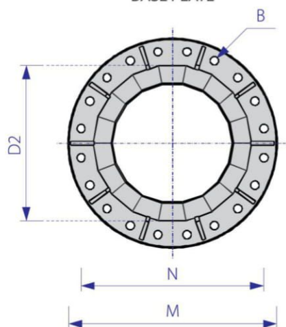
ĐỂ CỘT BASE PLATE
